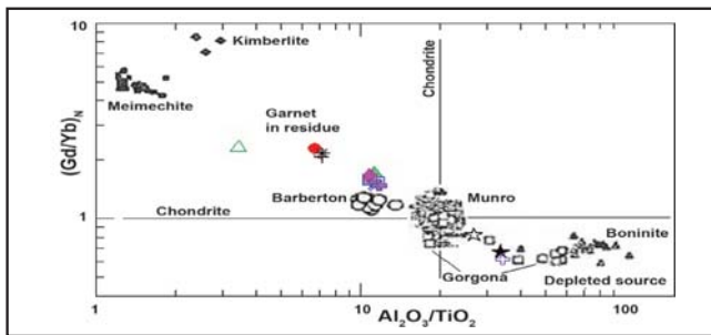
شکل ۱۲- نمودار Al_2O_3/TiO_2 در برابر (Gd/Yb)_N بهنجار شده بر حسب نسبت گوشته اولیه، موقعیت نمونه‌های فریمان در مقایسه با انواع کمانتیت‌ها در مناطق باربرتون، مونرو و گورگونا و دیگر سنگ‌های آتشفشانی غنی از MgO شامل میرمیکت‌ها، کیمبرلیت‌ها و بونیت‌ها، محدوده مجموعه‌های سنگی مختلف از (Arndt (2003). نمادهای رسم شده برای نمونه‌ها مانند شکل ۶.
